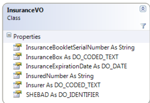
شکل ۶: - کلاس InsuranceVO
